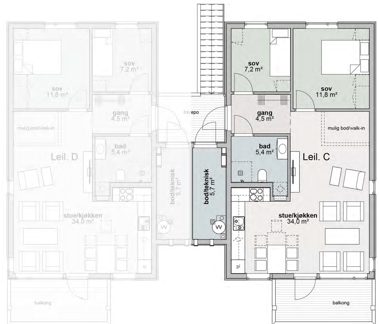
2. Etasje salgsplan 1 : 100
