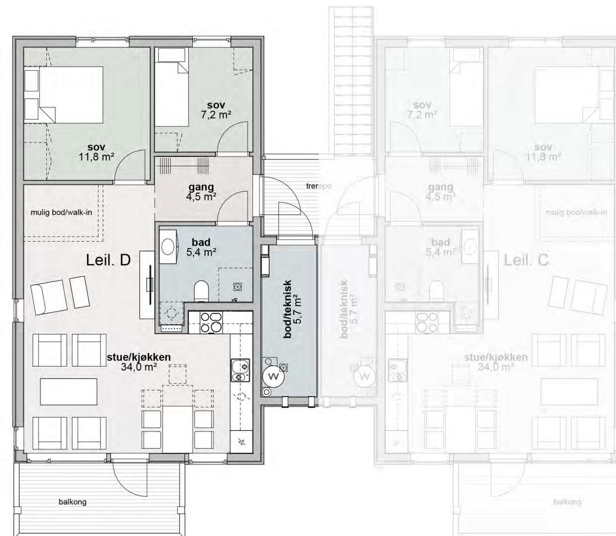
2. Etasje salgsplan 1 : 100
