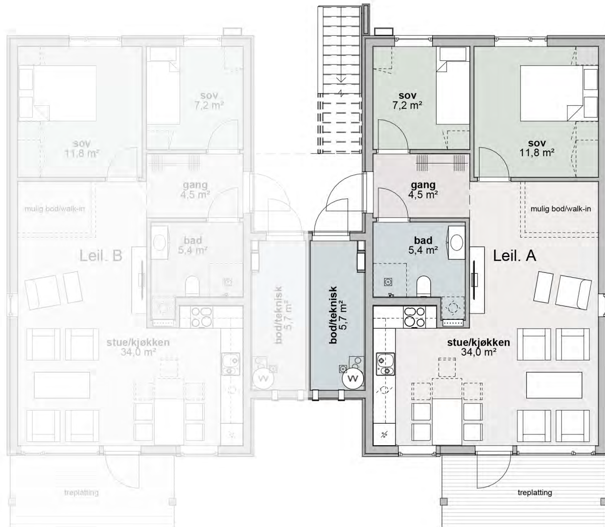
1. Etasje salgsplan 1 : 100
